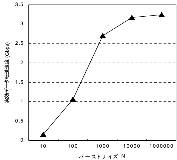
図5 バーストサイズNと実効転送速度
