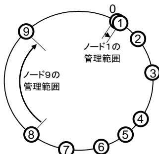
図1 ハッシュ空間内のノードの配置例
