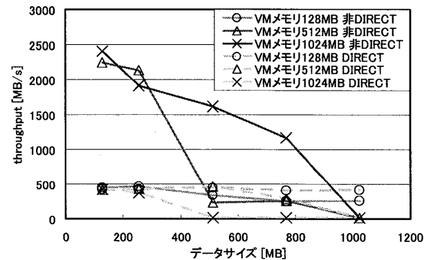
図 2 シーケンシャルリード測定結果
