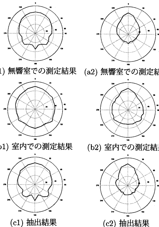
Fig 2: 方向ごとの放射指向特性の違いによるスピーカの音圧分布 (a1~c1: 2k Hz, a2~c2: 8 kHz)
