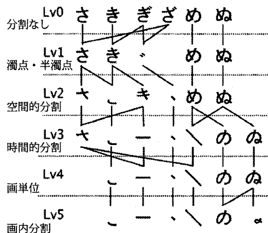
図 2: ひらがな用の文字構造辞書
