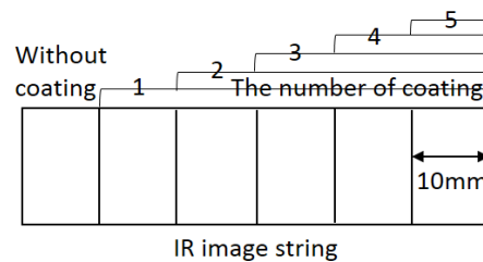
図11 赤外線画像の連結
