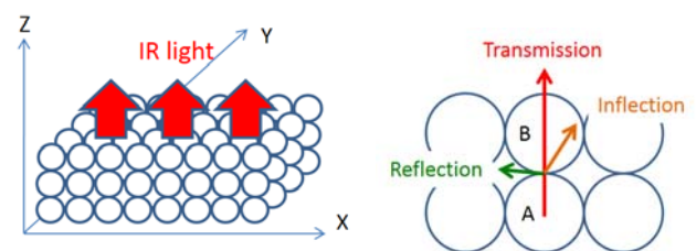
図5 (左) Z軸方向への発光の試み。
