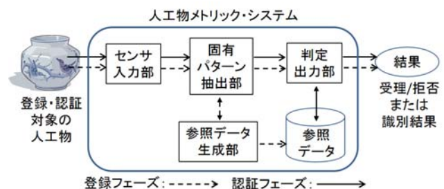
図1 人工物メトリック・システムの基本構成
