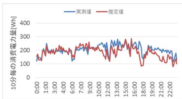
図 19 成分分離の検証結果(冷凍機) Figure 19 Separation test result (chilling unit)
