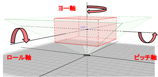
図2 Leap Motion の検知範囲
