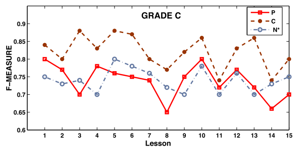
(d) Prediction results for grade C
