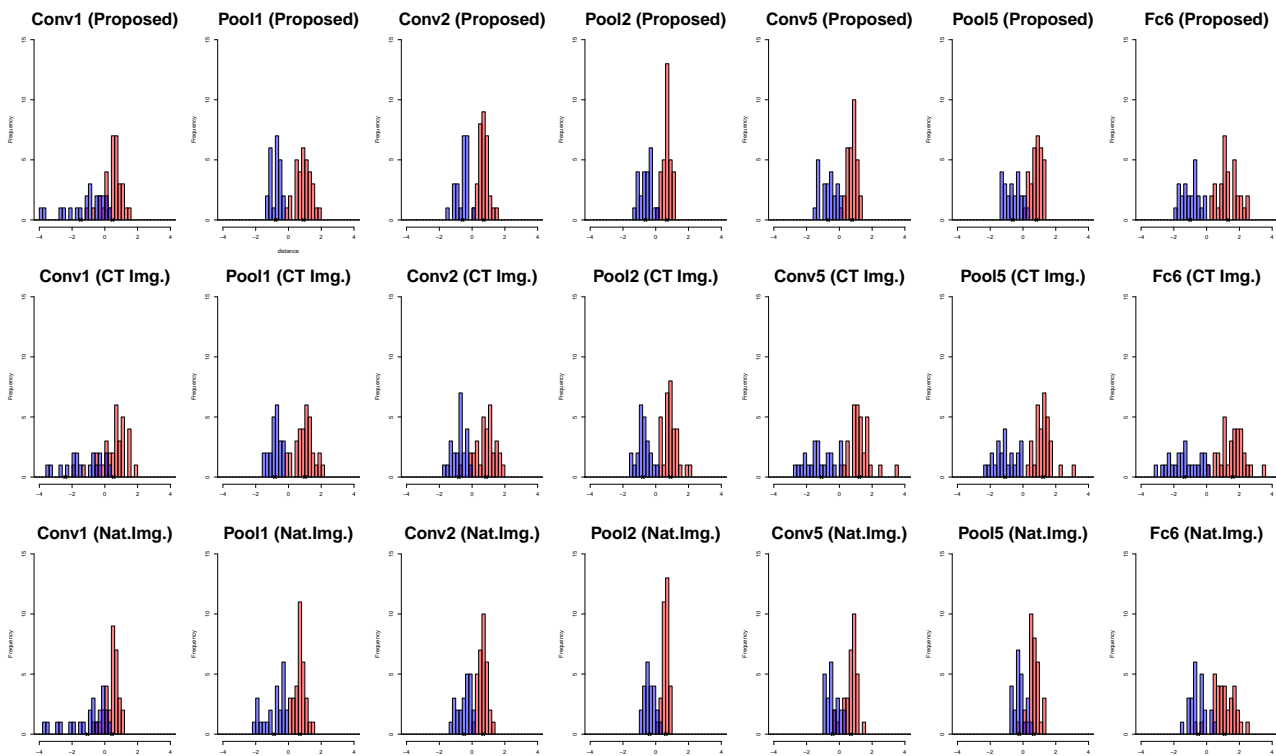
図 5 Nodular と GGO の 2 クラスにおける, SVM の分離超平面からの距離ヒストグラム. 右側のヒストグラムが Nodular, 左側のヒストグラムが GGO を示しており, それぞれ 1 と -1 がサポートベクトルの位置である. 各列は, 左から conv1 層, pool1 層, conv2 層, pool2 層, conv5 層 pool5 層, fc6 層で抽出した特徴を用いて学習したヒストグラムとなっており, 各段は, 上から提案手法, CT 画像のみ, 自然画像のみで学習したネットワークで抽出した特徴を用いている. 1, 3 段目の提案手法と自然画像を用いて学習した DCNN ではヒストグラムが階層を経るごとに徐々に細くなっている事が見て取れる.
