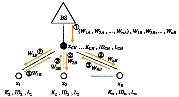
図 2.提案方式 2 の鍵共有方式
