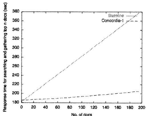
図 4 適合する上位文書の収集時間
