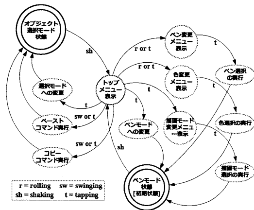
図 2: Oh! Stylus Draw 3 の操作体系
