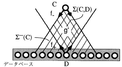
図 6 上と下からの探索を用いた g' の導出 Fig. 6 Generation of g' from g by f_- and f_+ algorithms.
