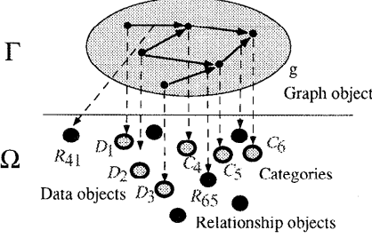
図4 階層構造グラフモデルのレイヤー構造 Fig. 4 Two-layered structure for hierarchical graphs.
