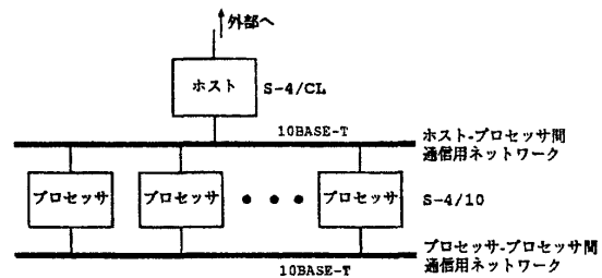
図1: マシン間接続図
