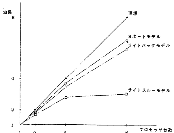
図1 台数効果
