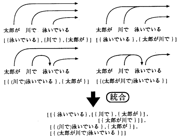
図1: 「太郎が川で泳いでいる...」のスタック表現
