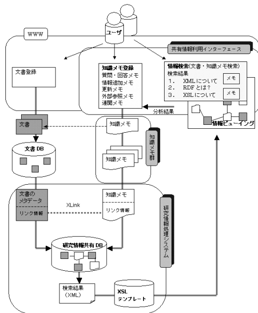
図1 システム全体図
