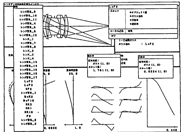
図2 レンズ設計支援システムの実行例
