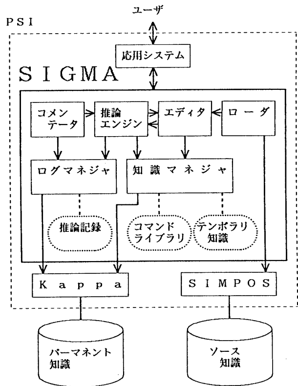
図1 SIGMAのシステム構成
