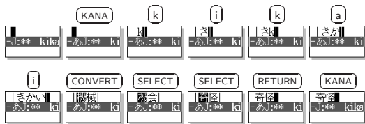
図 3 「奇怪」をかな漢字変換で入力 Fig. 3 Kana-Kanji conversion for 「奇怪」.
