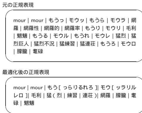
図 7 “mour” に対する正規表現の最適化 Fig. 7 Optimization of the regular expression for “mour”.
