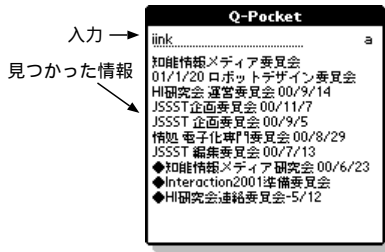
図 11 個人情報のインクリメンタル全文検索
