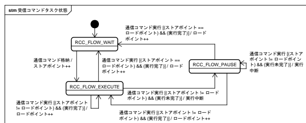
図 4 通信コマンド実行タスク状態遷移図
