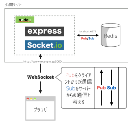
図 11 本システムの構成図
