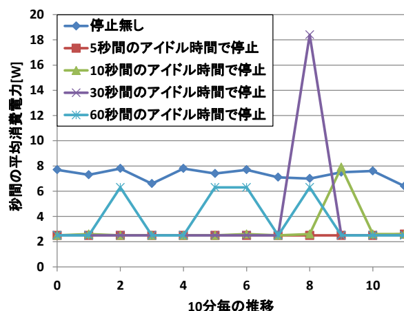
図 13 停止設定による電力の推移
