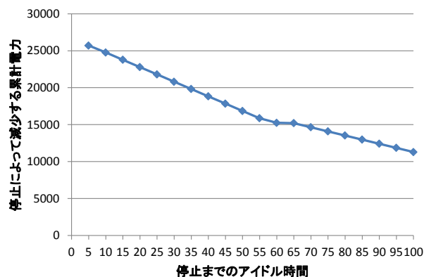
図10 停止によって減少する累計電力と アイドル時間の関係図
