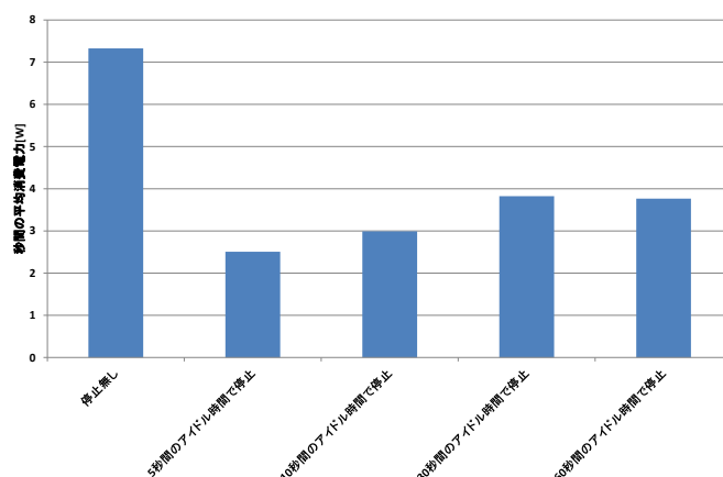
図 12 停止時間による平均消費電力
