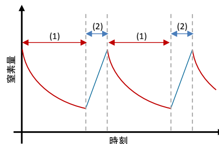
図 8 給液タンク内室素量の遷移
