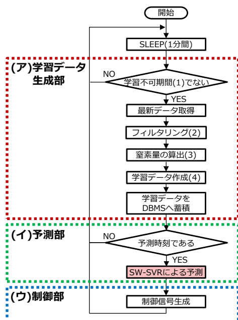
図 7 知的システムフローチャート
