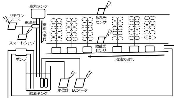
図 6 各種センサ配置図
