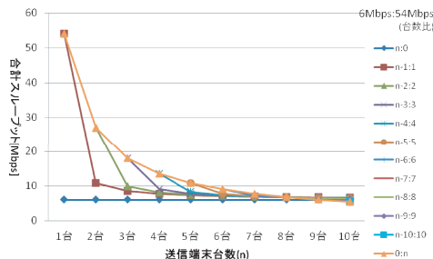
図 2: 近似式におけるスループット
