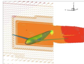
図 1 : 圧力・流速分布可視化例
