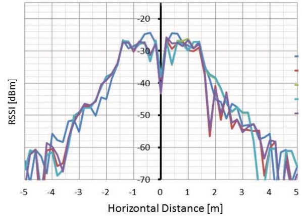
図 25 シミュレーション結果 (直線配置) Fig. 25
