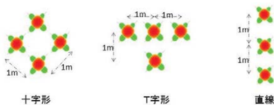
図 24 アンテナ配置 Fig. 24 Antenna layout of each antenna array
