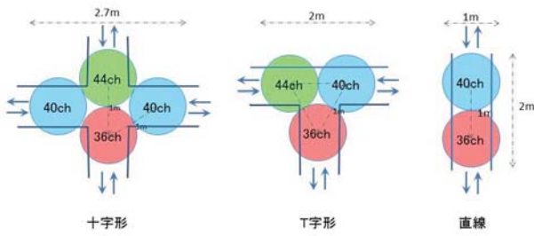
図 22 複数のチャンネルを使用する Wi-Fi ビーコンアレイ Fig. 22 Channel assign of the Wi-Fi beacon arrays
