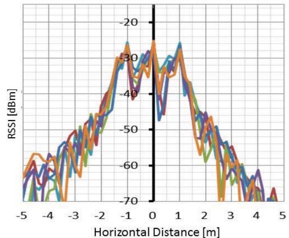
図 26 シミュレーション結果 (T 字形配置) Fig. 26
