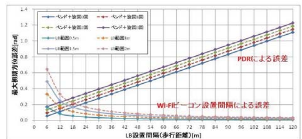
図 31 Wi-Fi ビーコンの設置間隔と PDR 誤差の関係 Fig. 31 Trade off of the Errors
