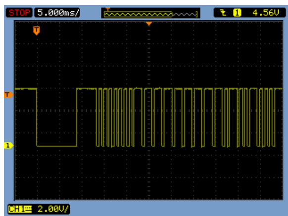
図5 CH1のNEC送信フォーマット
