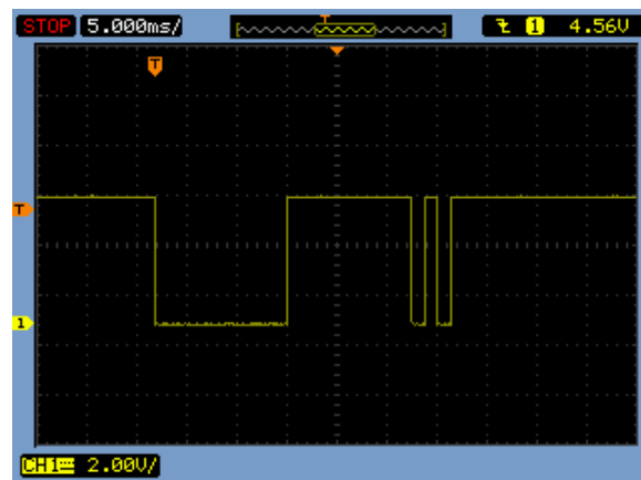
図6 サンプルプログラムの出力波形 Figure 6 Output Waveform of A Sample Program.
