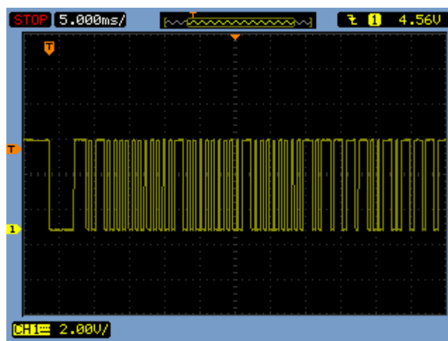
図10 CH1の出力波形
