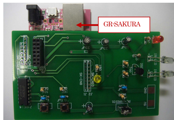
図3 使用したマイコンボードと結合 Figure 3 Combination of IR-Transceiver Board and GR-SAKURA Board.
