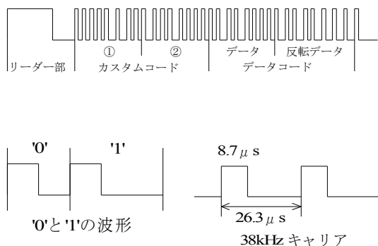
図8 NEC送信フォーマット
