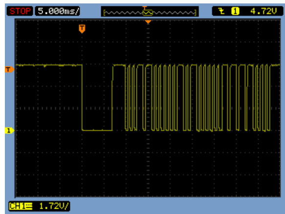
図 12 「前進」ボタンのリモコン波形
