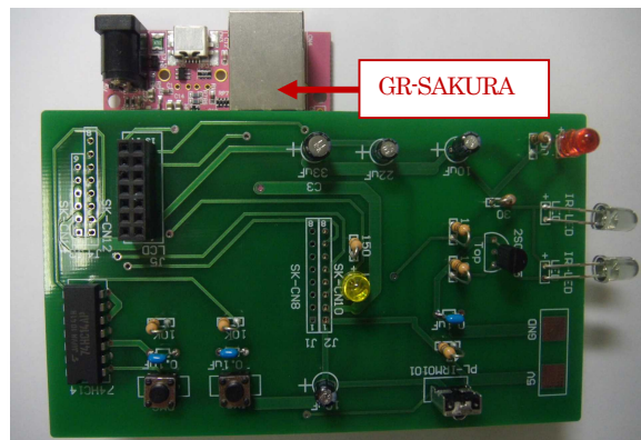
図3 使用したマイコンボードと結合 Figure 3 Combination of IR-Transceiver Board and GR-SAKURA Board.
