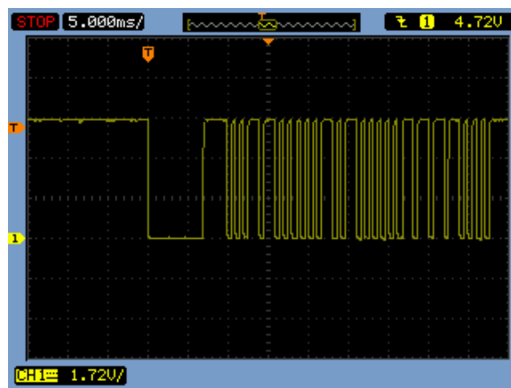
図 12 「前進」ボタンのリモコン波形
