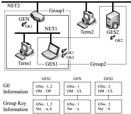
図 3 ネットワーク構成図と GE 定義情報 Fig. 3 Network model and GE definition information.
