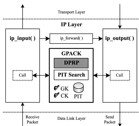
図 6 GSCIP の実装 Fig. 6 Implementation of GSCIP.
