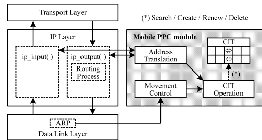
図 7 モジュール構成 Fig. 7 Module structure.
