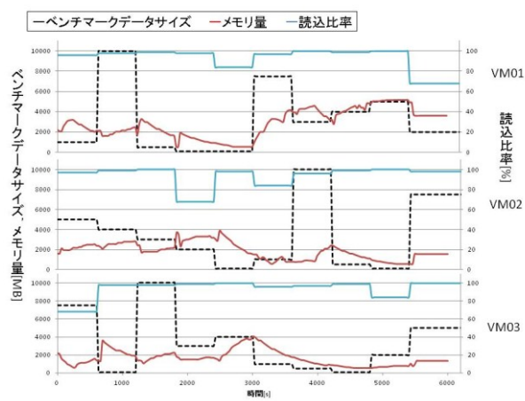
図19 ベンチマークデータサイズとVMのメモリ量の関係 ( \alpha=25 )
