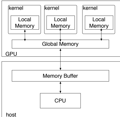
図 4 Gpu Architecture
