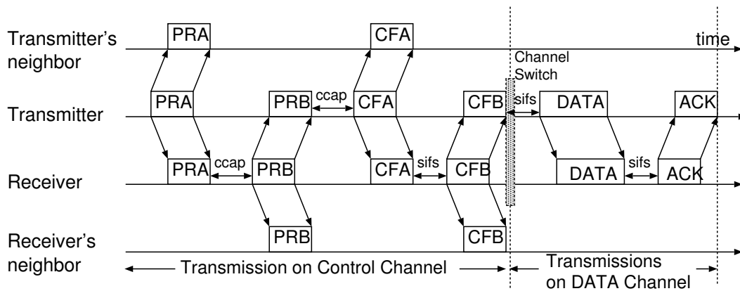
図 2 CAM-MAC の動作
