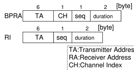
図 5 B-MAC のフレームフォーマット
