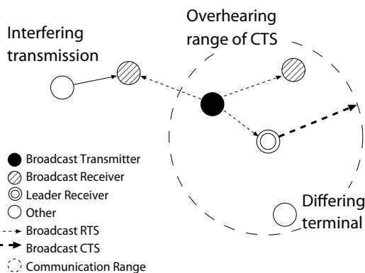
図 3 LBP の動作
