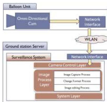
図2. システムアーキテクチャ
