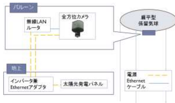
図 8. バルーンに搭載する機器構成
