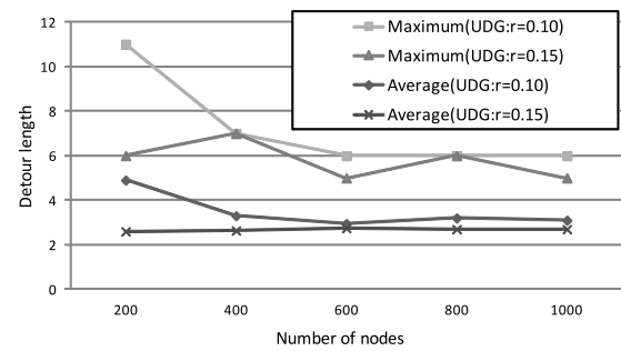
Fig. 14 Detour path length on UDG.
